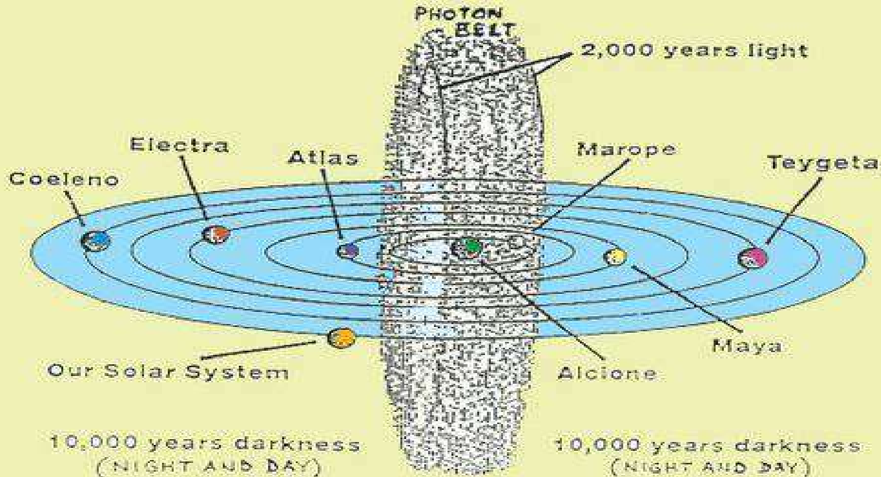
The Pleiades
